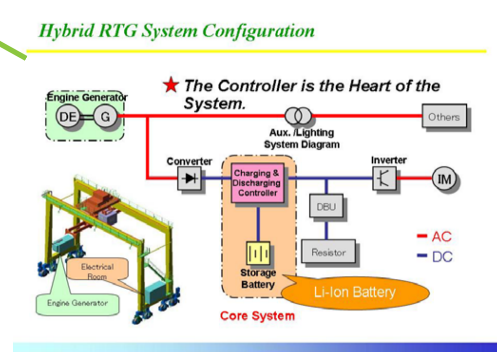
混能龍門吊機運作原理 Hybrid RTG System Configuration
