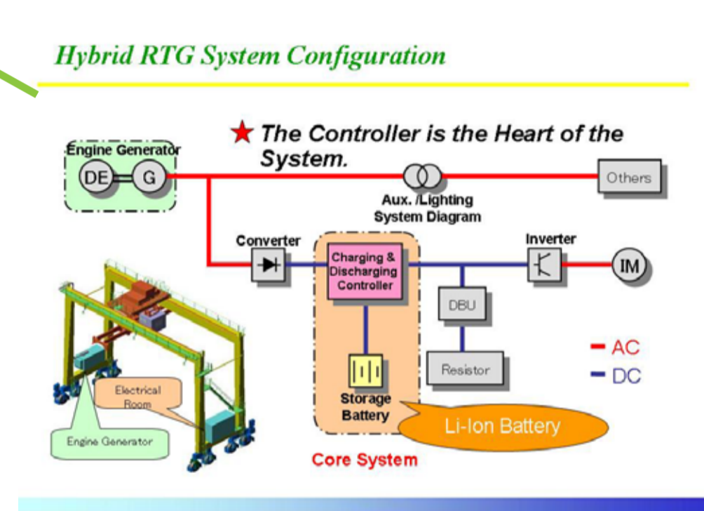
混能龍門吊機運作原理 Hybrid RTG System Configuration
